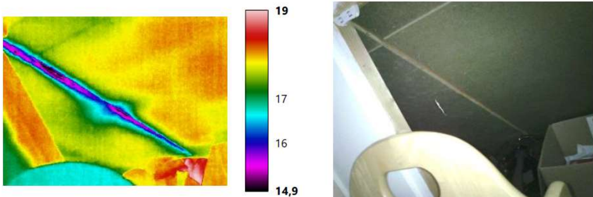
Beeld van warmteverlies/ luchtlekkage langs dakplaten..
